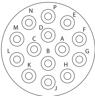
Socket
