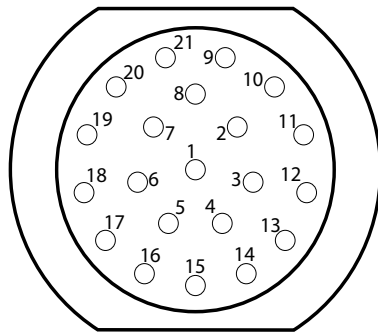
1625 Deutsch HDP24-18-21PN
