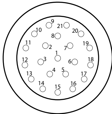
1619 Deutsch HDP26-18-21SN
